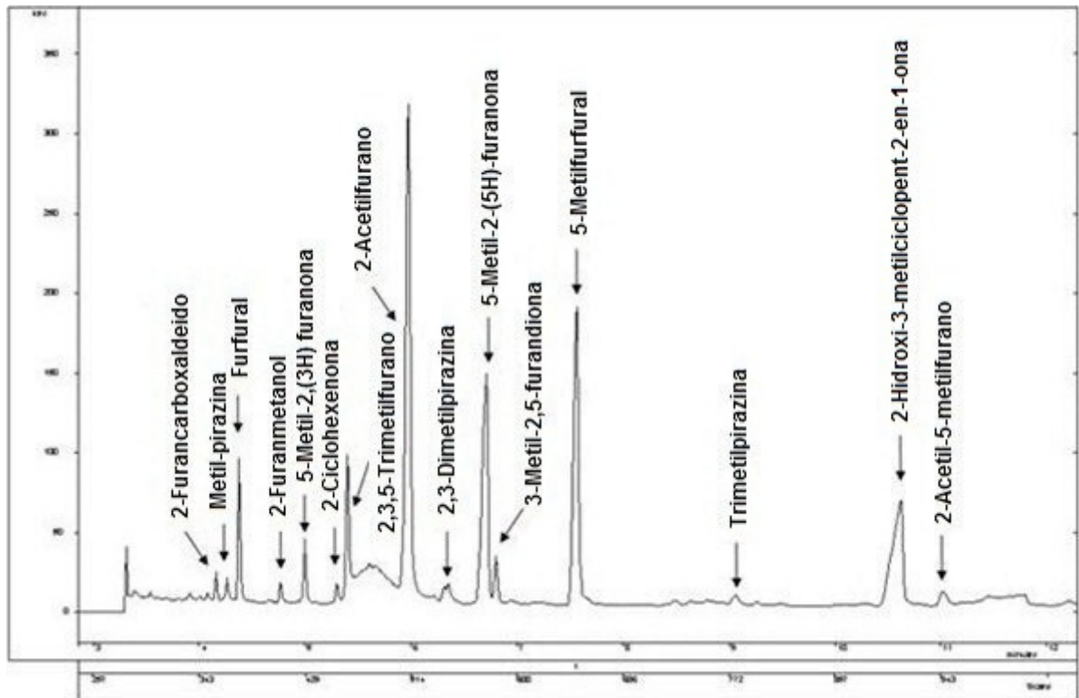
Figura 4. Cromatograma do corante caramelo Classe IV da marca A
